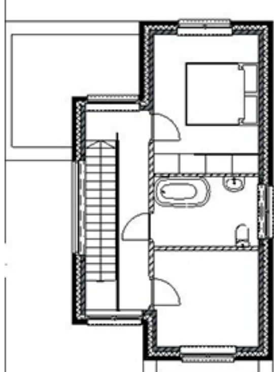
Grondplan Verdieping 2
