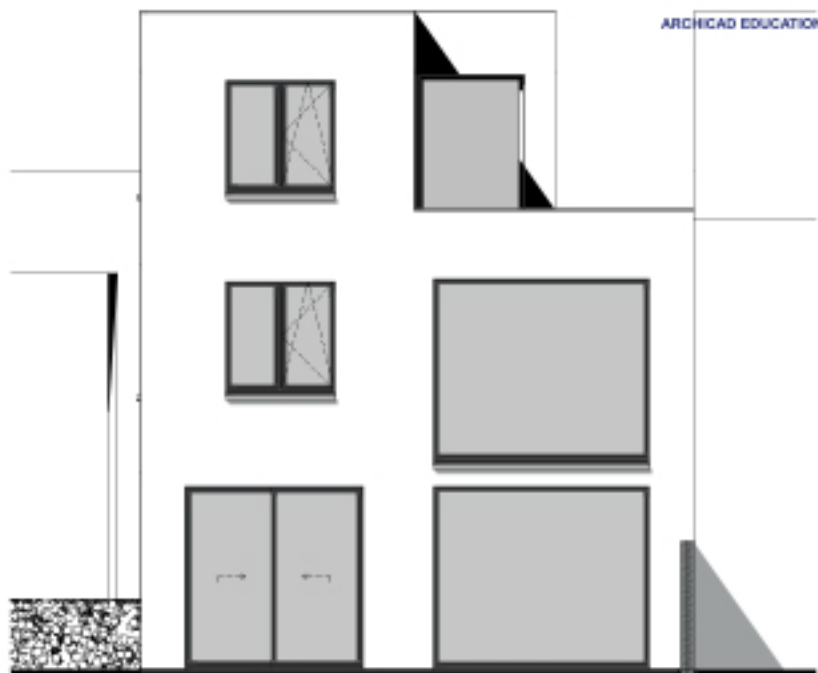
Achtergevel
