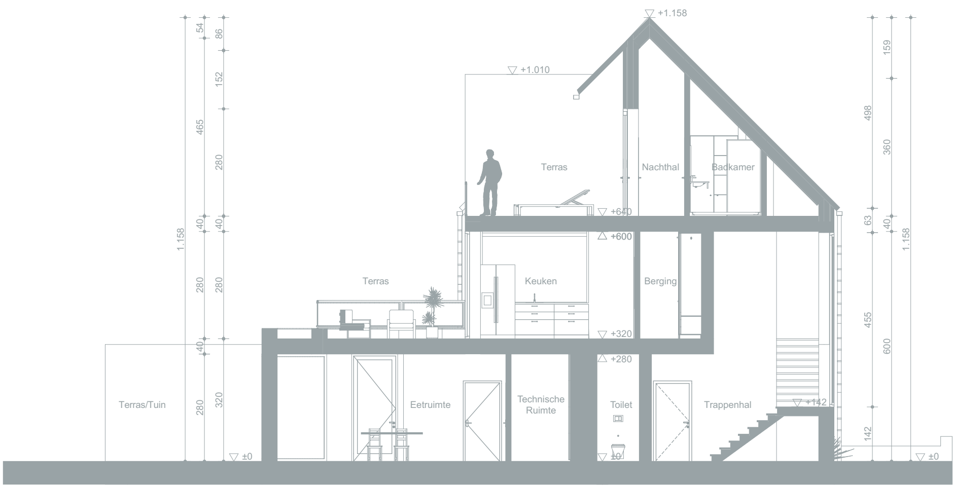
Snede A-A 1/100
