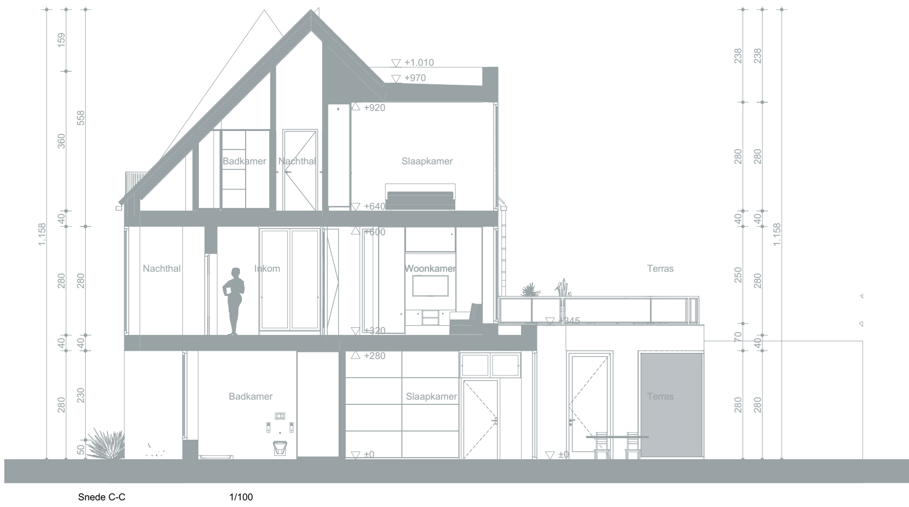
Snede C-C 1/100
