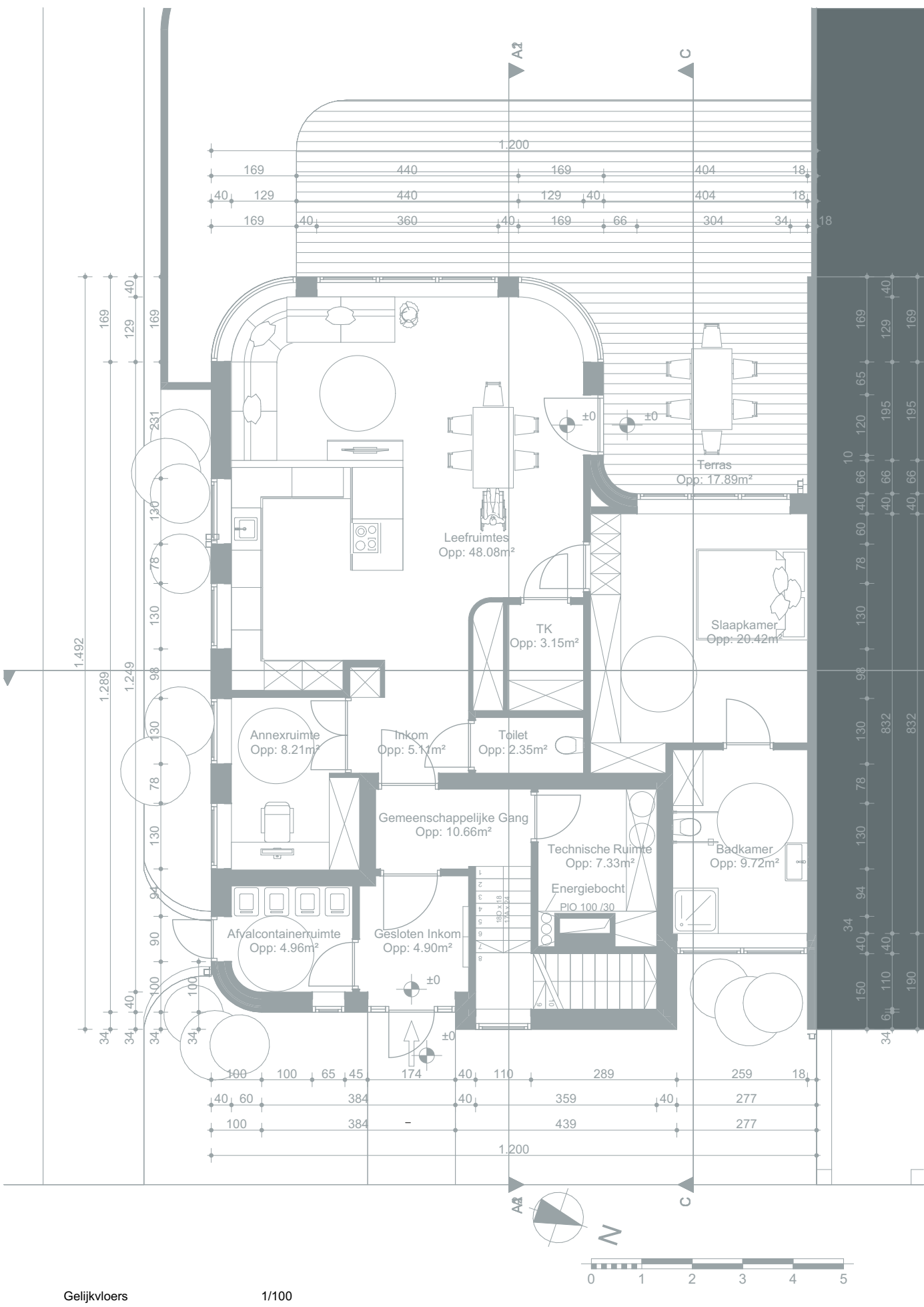
Gelijkvloers 1/100
