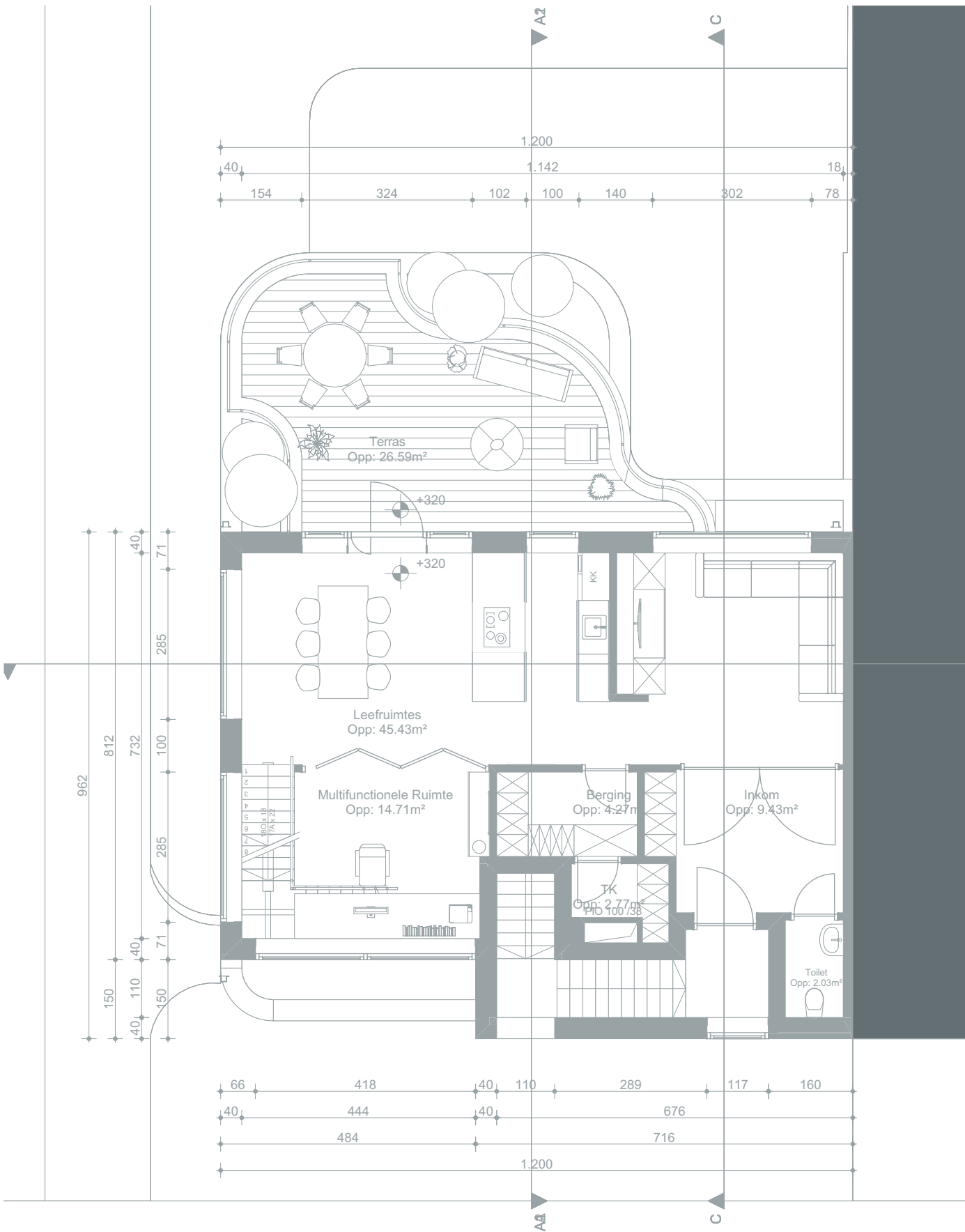
Verdieping 1 1/100
