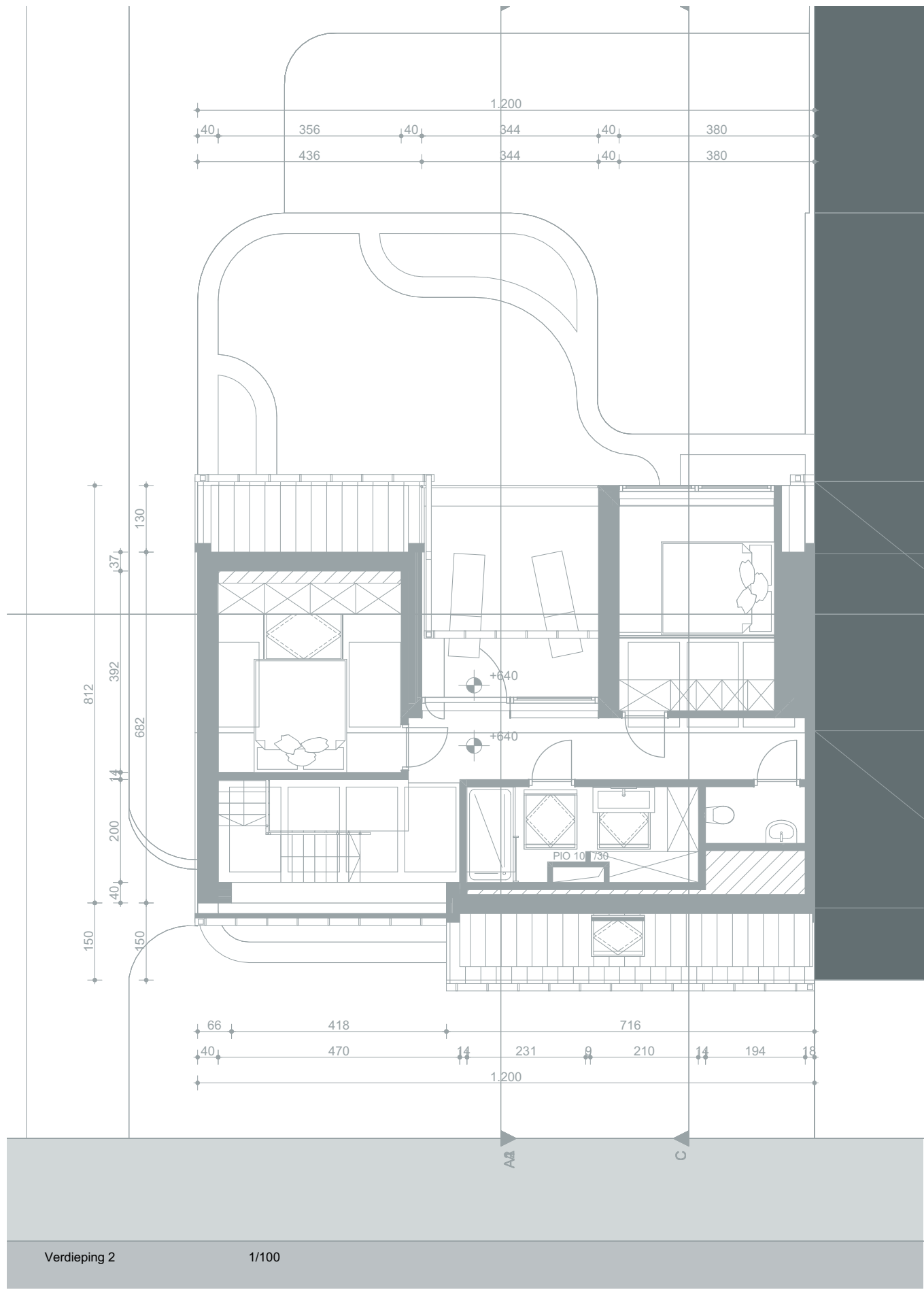
Verdieping 2 1/100
